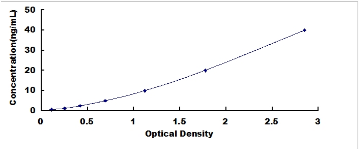
小鼠胱天蛋白酶 3 (CASP3) 检测试剂盒标准曲线
